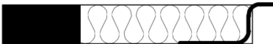
System 2: Vorkomprimiertes Dichtungsband, PU-Schaum oder Stopfwollzopf (Hanno®-Zopf), Folienband FI, Folienband Duo Easy 240
