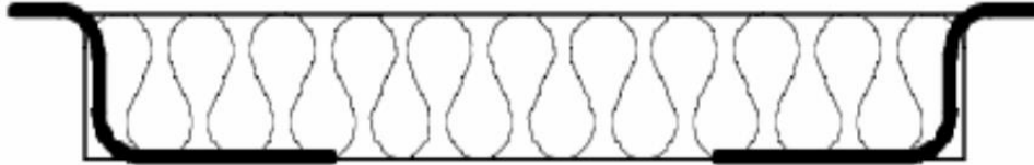
System 3: Folienband FA oder DUO Easy, PU-Schaum oder Stopfwole (Hanno®-Zopf), Folienband FI oder DUO Easy
